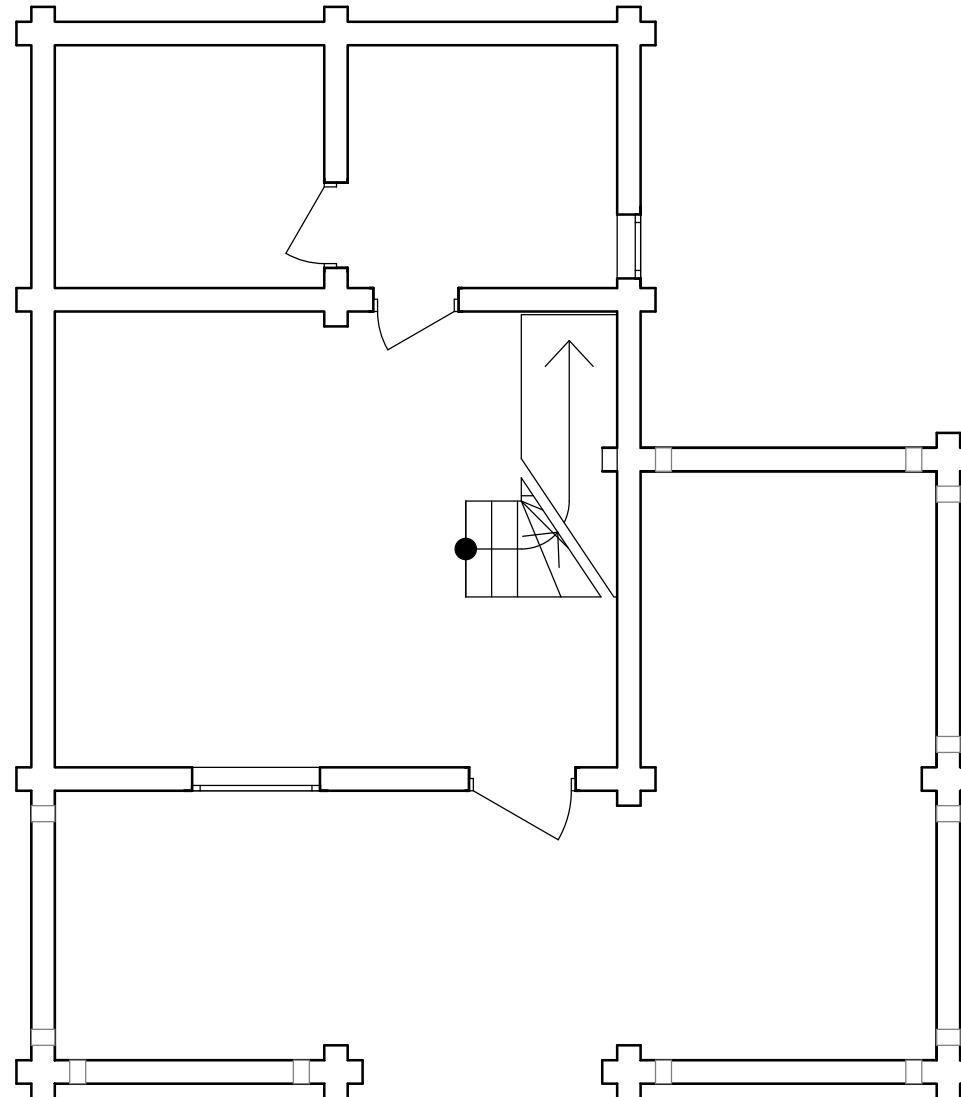
План сруба
