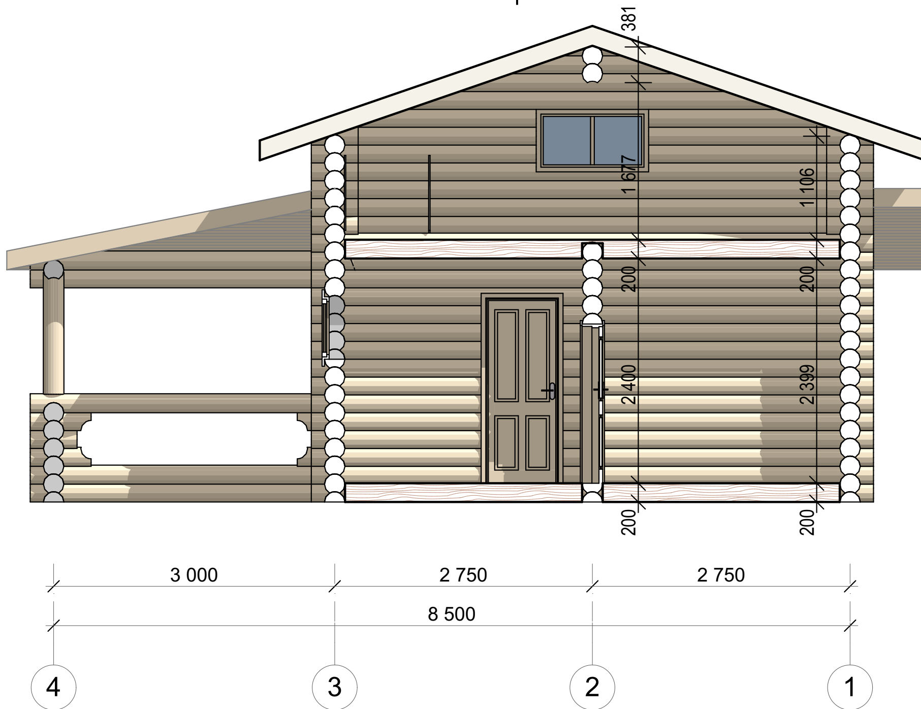
Разрез 2-2
